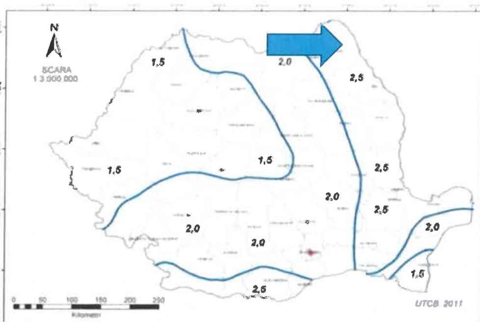
Fig.3 – Zonarea Teritoriului din punct de vedere al înălțării din zăpadă
